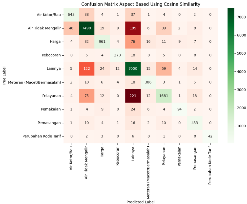
Gambar 4. 5. Confusion Matrix Skenario 2 Percobaan Pertama
